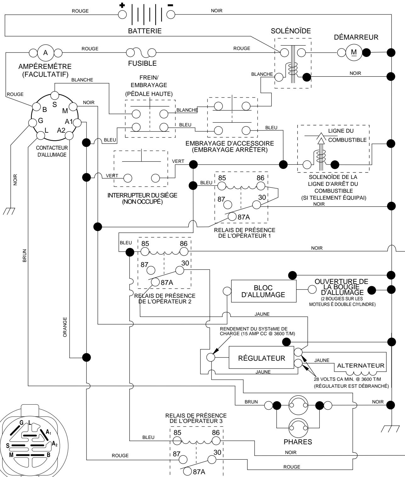
CONTACTEUR D'ALLUMAGE
