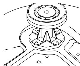
MANDRIN DE CARTER DE STYLE "B"
