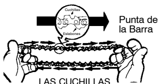
LAS CUCHILLAS DEBERAN APUNTA EN DIRECCION A LA ROTACION
