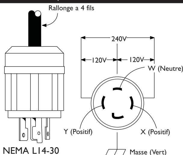
Figure 18 – Prise à Verrouillage de 120/240 Volts c.a., 30 Ampères
