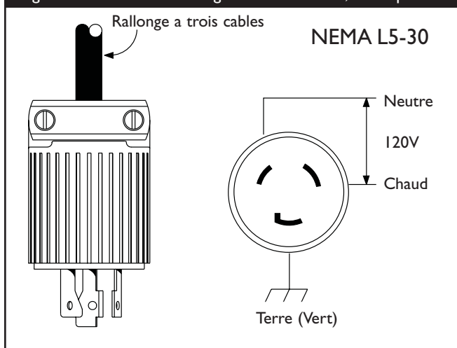
Figure 19 - Prise à Verrouillage de 120 Volts c.a., 30 Ampères
