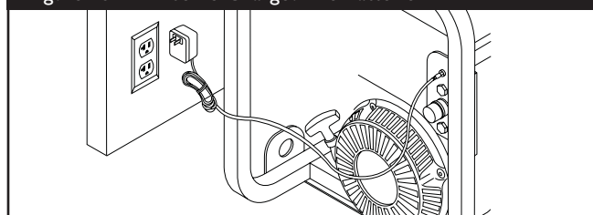
Figure 15 — Prise de Chargeur de Batterie
