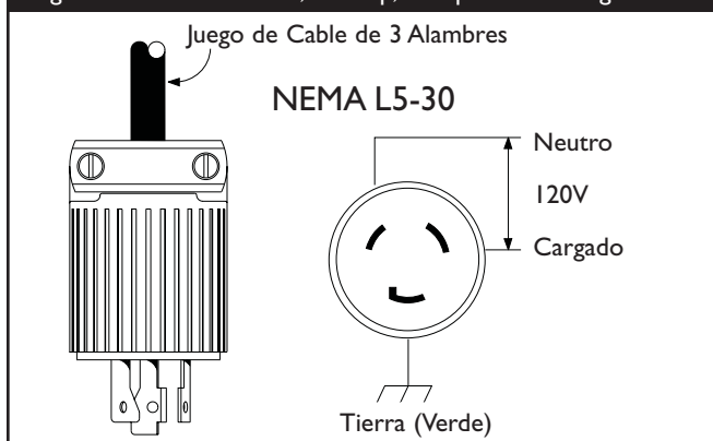
Figura 30 — 120 Volt AC, 30 Amp, Receptáculo de Seguridad
