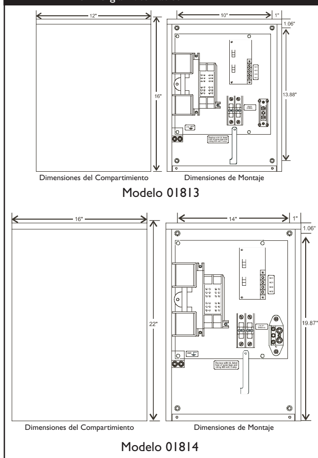
Figura 7 — Dimensiones del Conmutador de Transferencia de Energía Automático
