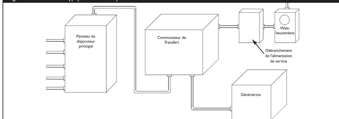
Figure 5 — Installation Typique d'un Interrupteur
