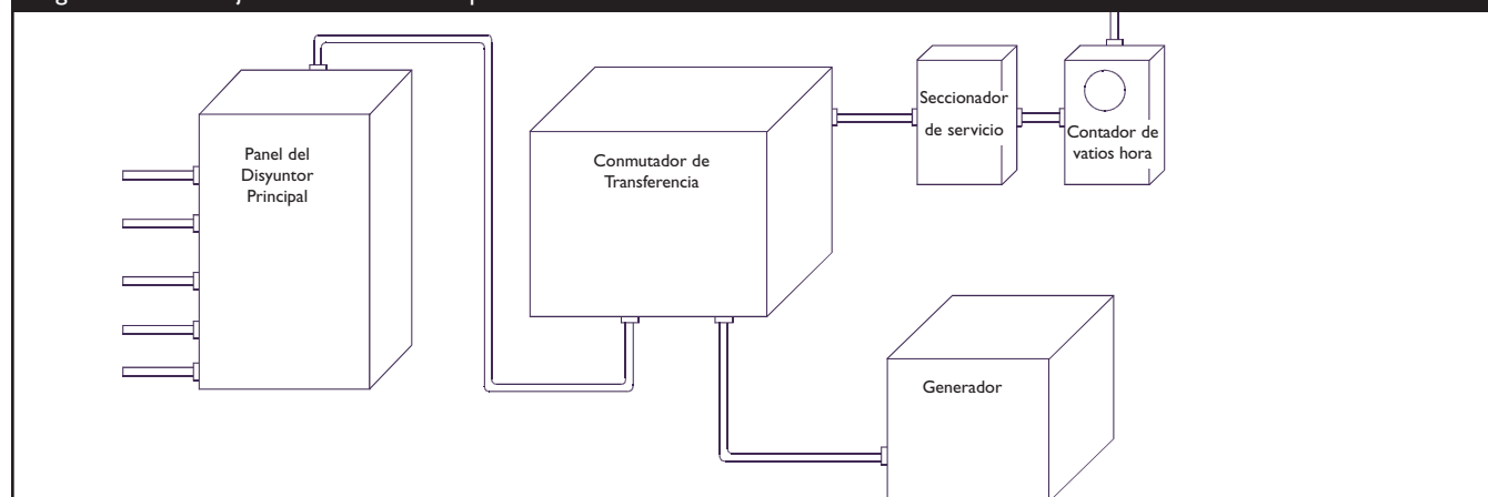
Figura 8 — Montaje del Conmutador Típico
