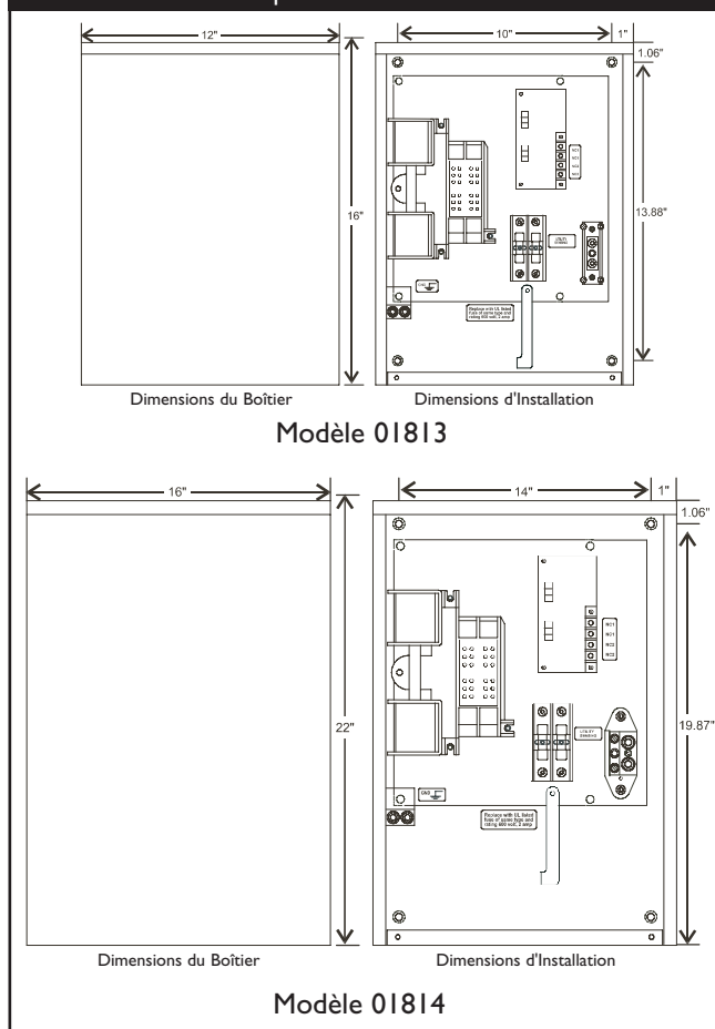
Figure 4 — Dimensions du Commutateur de Transfert Automatique
