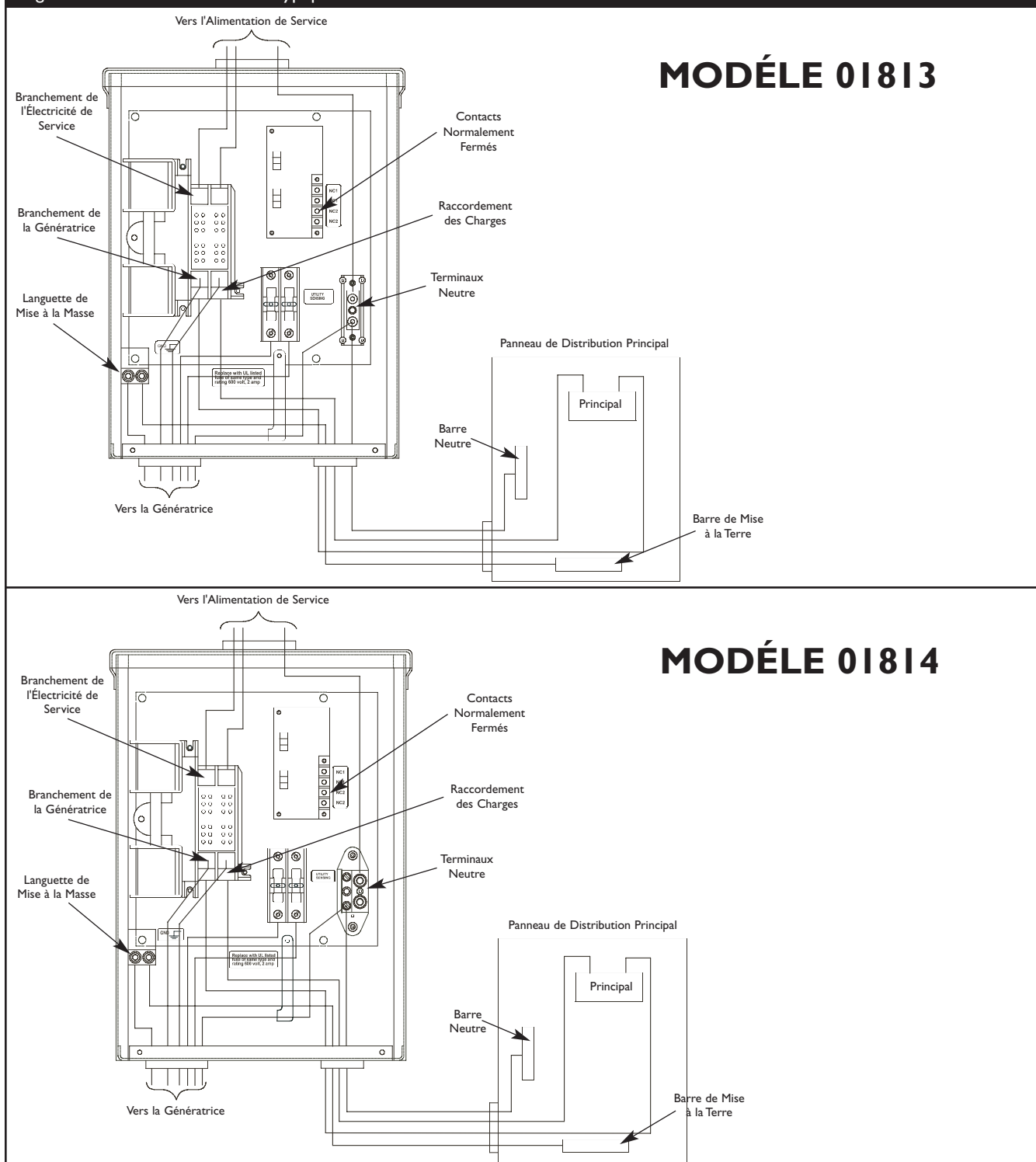
Figure 6 — Schéma d'Installation Typique du Commutateur de Transfert
