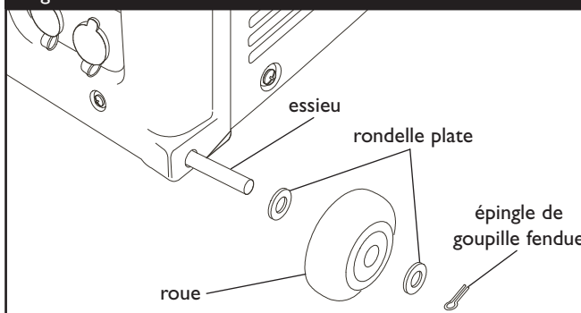
Figure 16 — Installation de l'ensemble de roues
