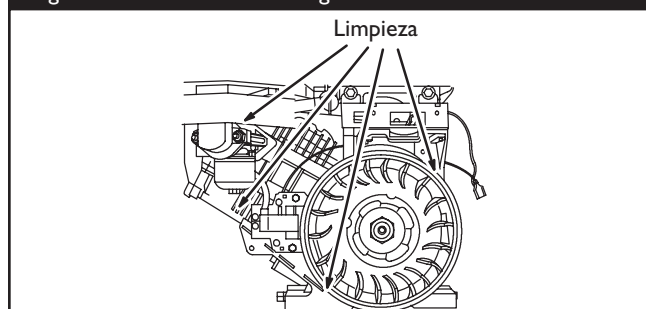
Figura 51 — Sistema de Refrigeración de Aire
