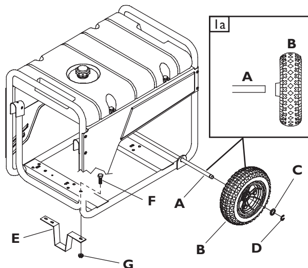
Figura 1 — Instale el Juego de Ruedas
