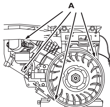
Figura 15 — Sistema de Refrigeración de Aire A - Limpie estas Áreas
