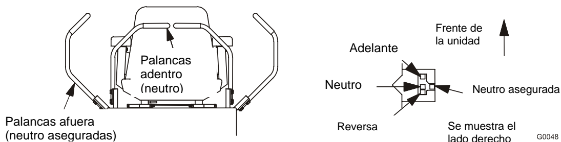
FIGURA 2 POSICION DE LAS PALANCAS DE MOVIMIENTO
