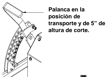
FIGURA 5 POSICION DE ALTURA DE CORTE
