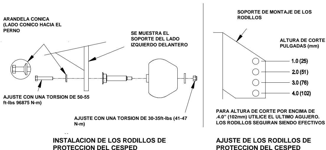
FIGURA 6 AJUSTE DE LOS RODILLOS
