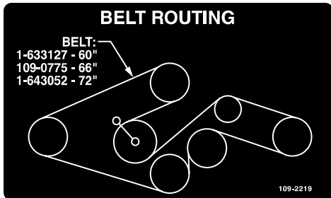
Nº de PARTE 109-2219 UBICACION: Bajo el posa pies, en la plataforma de corte.
