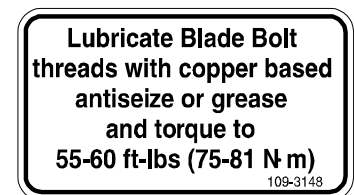
PARTE NO. 109-3148 UBICACION: Lado izquierdo al frente de la plataforma de corte
