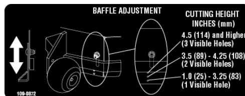
Nº de PARTE 109-0872 UBICACION: Lado izquierdo de la plataforma de corte.
