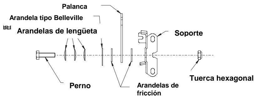
FIGURA 11 TENSION DEL ACELERADOR
