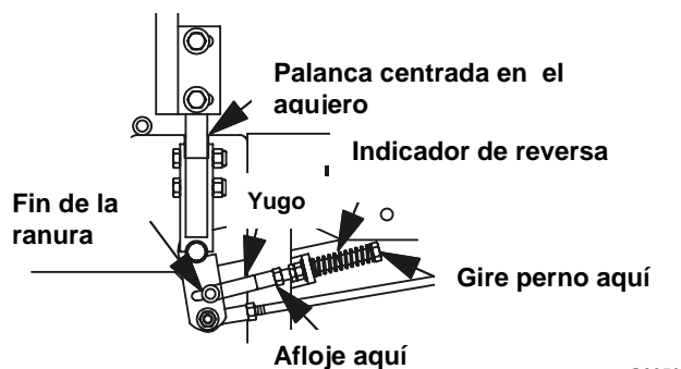
FIGURE 12 AJUSTE DEL INDICADOR DE REVERSA
