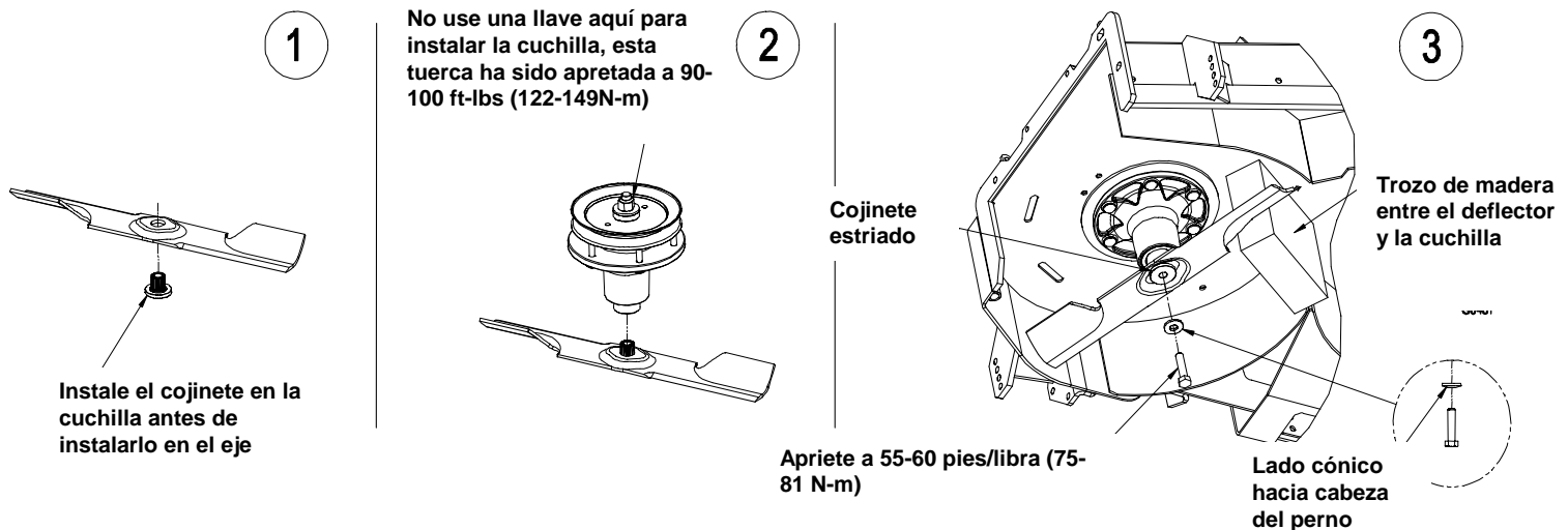
FIGURA 3 INSTALACION DE LA TUERCA DE LA CUCHILLA
