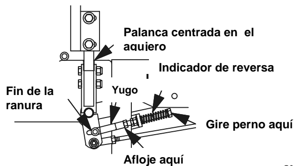
FIGURE 13 AJUSTE DEL INDICADOR DE REVERSA
