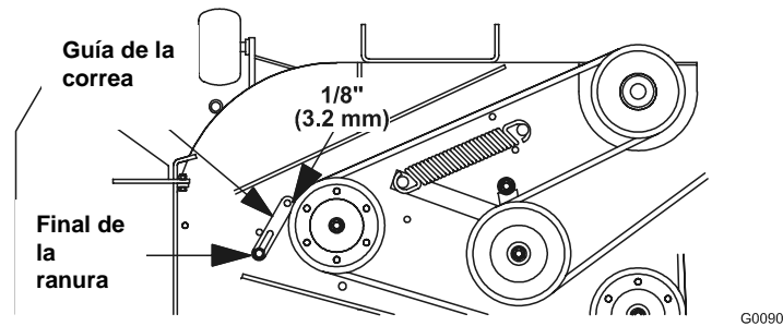
FIGURA 10 POSICION DE LA GUIA DE LA CORREA
