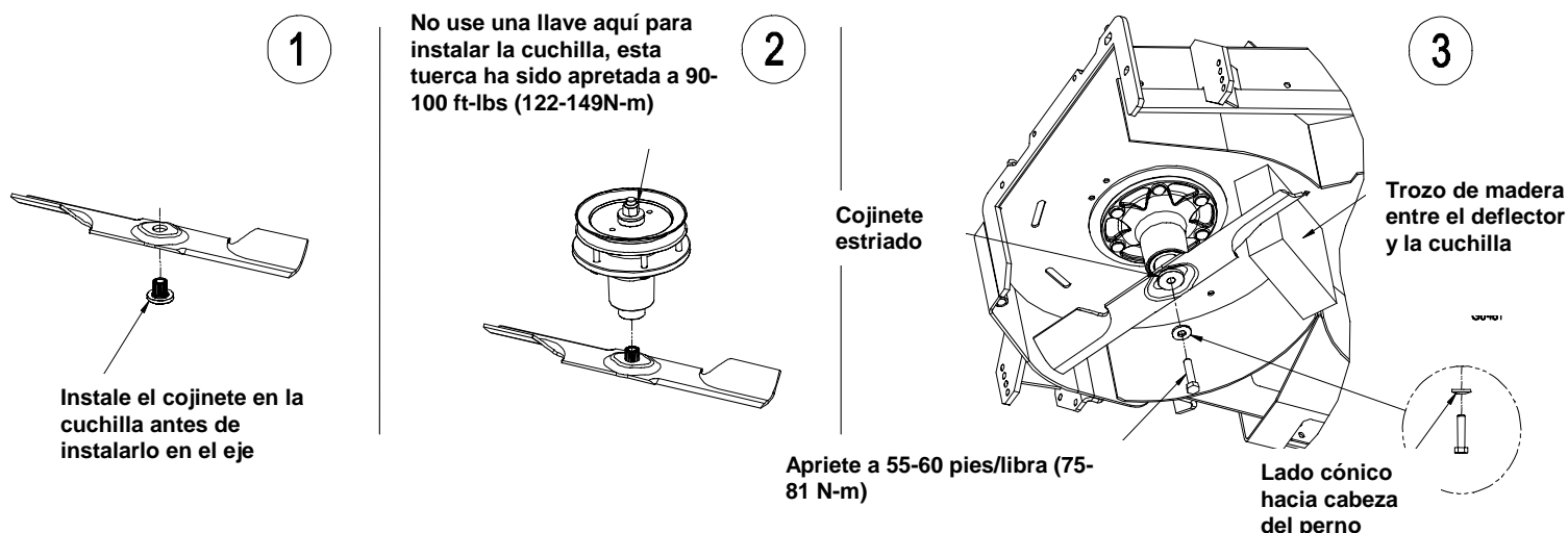
FIGURA 3 INSTALACION DE LA TUERCA DE LA CUCHILLA
