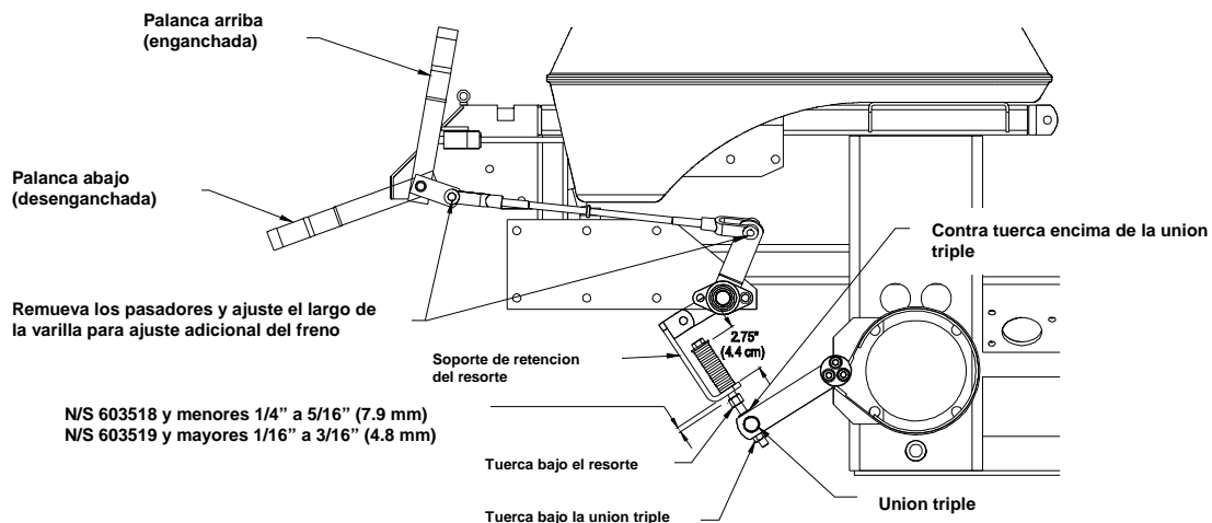
FIGURE 10 AJUSTE DEL FRENO
