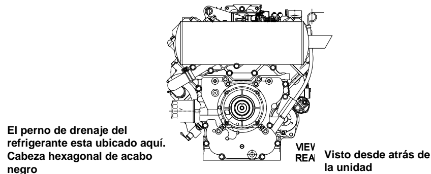
FIGURA 8 UBICACIÓN DE LA TUERCA DE DRENAJE DEL REFRIGERANTE
