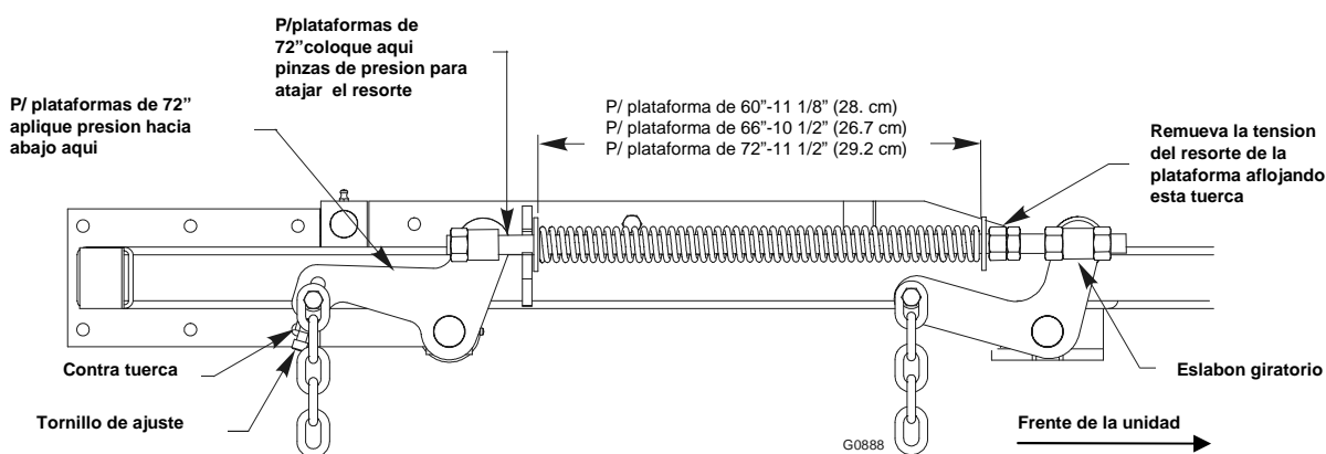
FIGURE 7 AJUSTE DEL ESLABON GIRATORIO AJUSTE DE TENSION DE LOS RESORTES DE LA PLATAFORMA
