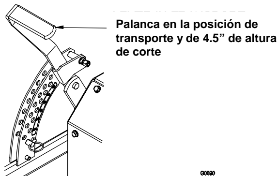
FIGURA 5 POSICION DE ALTURA DE CORTE
