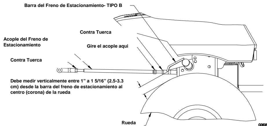
FIGURA 9 TIPO B – AJUSTE DEL FRENO DE ESTACIONAMIENTO
