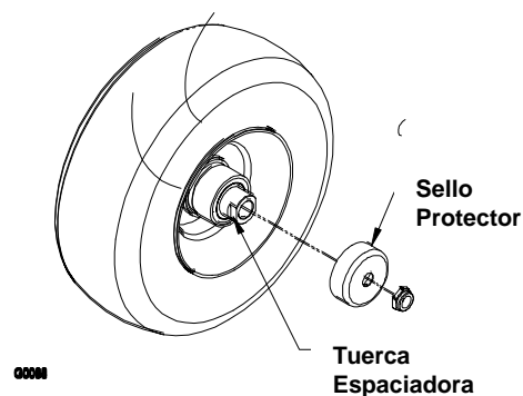
FIGURA 4 ENSAMBLE RUEDA DELANTERA
