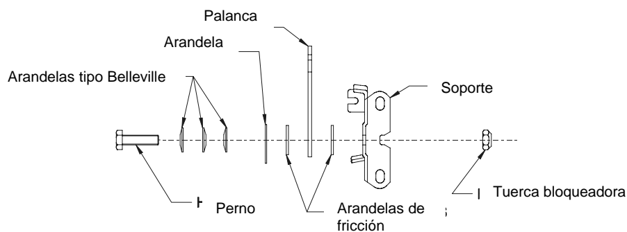
FIGURA 9 TENSION DEL ACELERADOR
